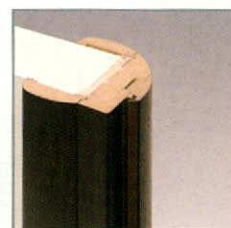
Finishing of Arcus door frame: moulding 19x60mm коробка Arcus - Отделка: наличник 19x60 мм Toc Arcus - pervaz 19 x 60 mm каса Arcus - Декоративен перваз 19x60 мм Arcus ajtótok - szegőléc 19x60mm
